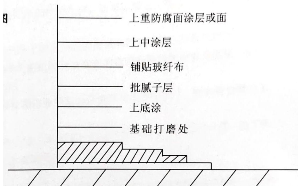
图 7.9-1 本项目防腐围堰施工结构图
