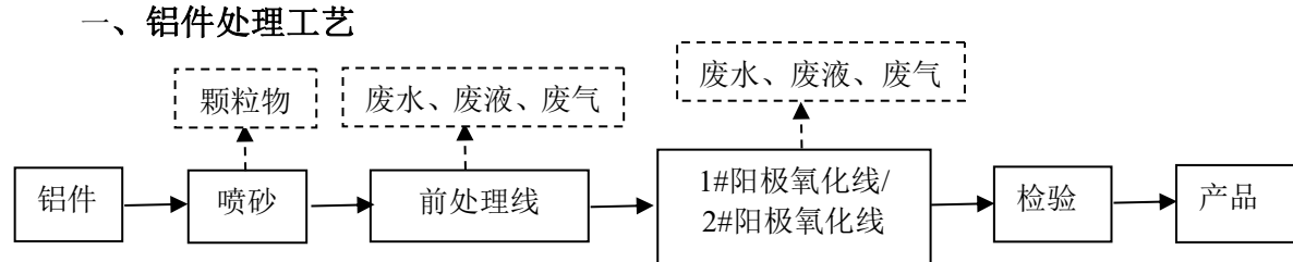
图 4.1-1 项目生产工艺流程图
