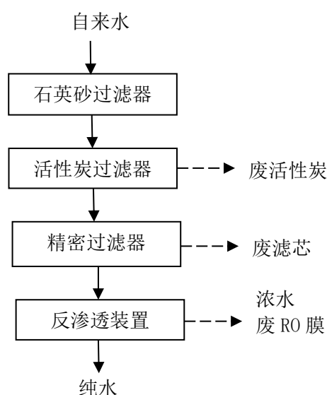
图 4.1-5 纯水制备工艺流程及产污环节图
