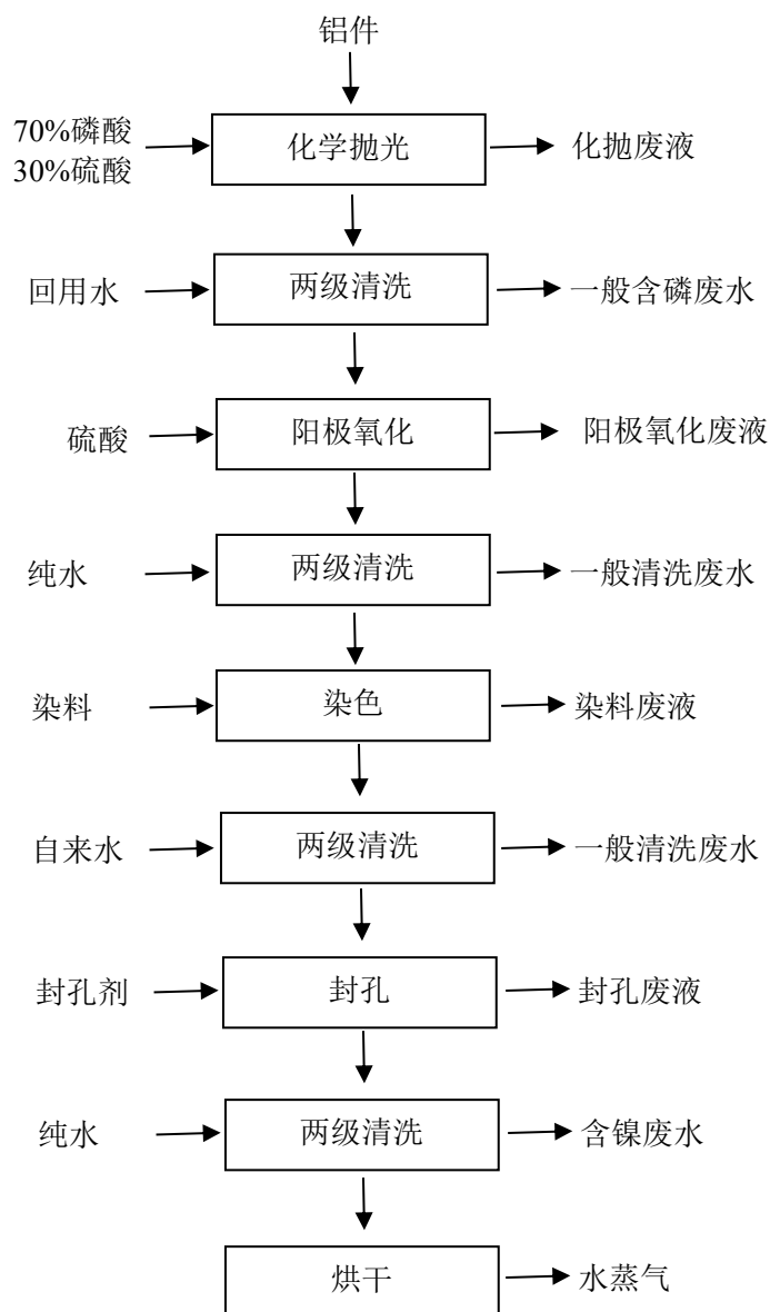
图 4.1-3 1#阳极氧化线工艺流程及产污环节图
