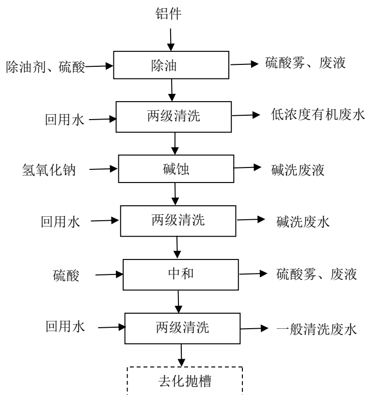
图 4.1-2 前处理线工艺流程及产污环节图
