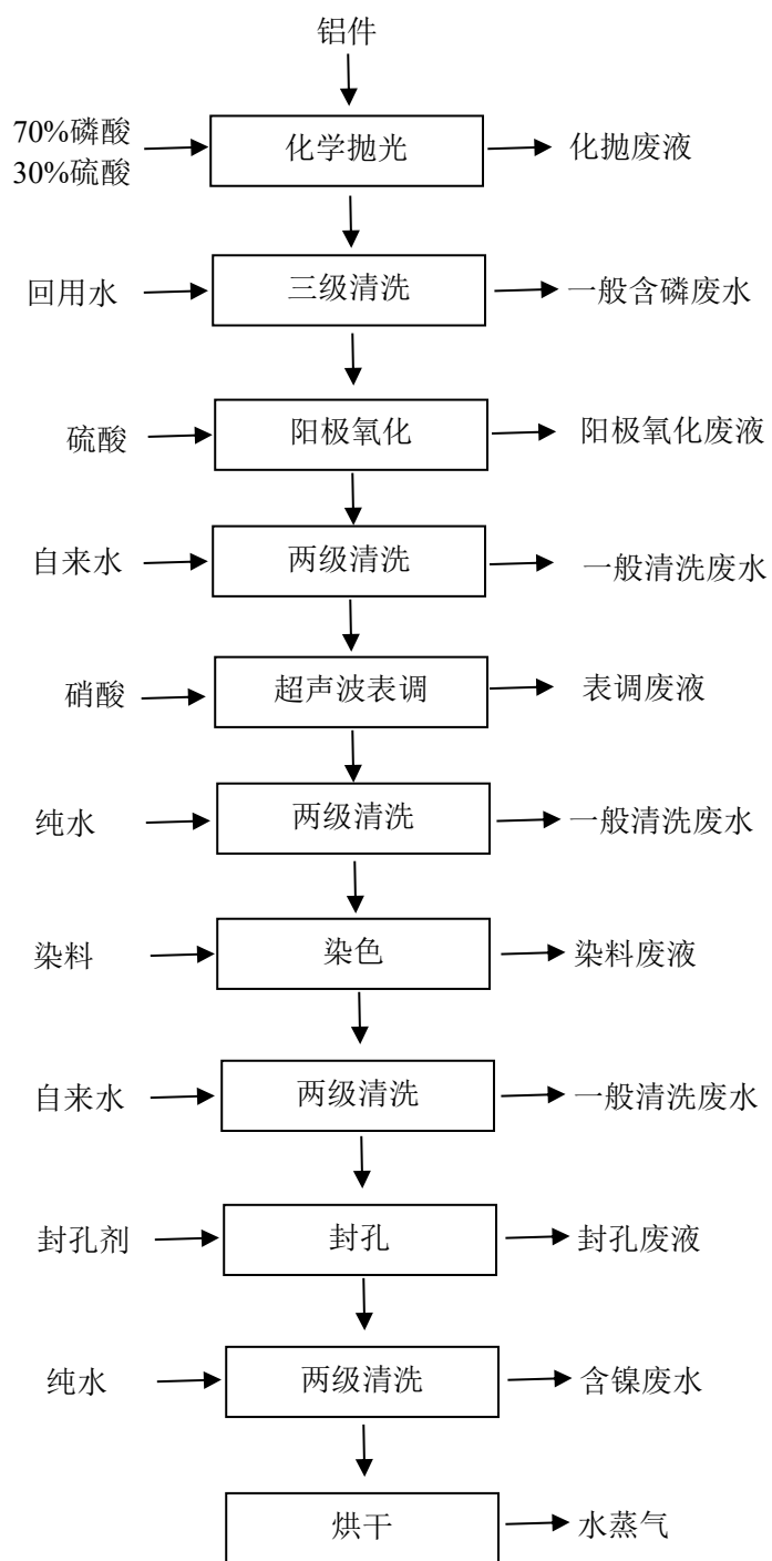
图 4.1-4 2#阳极氧化线工艺流程及产污环节图
