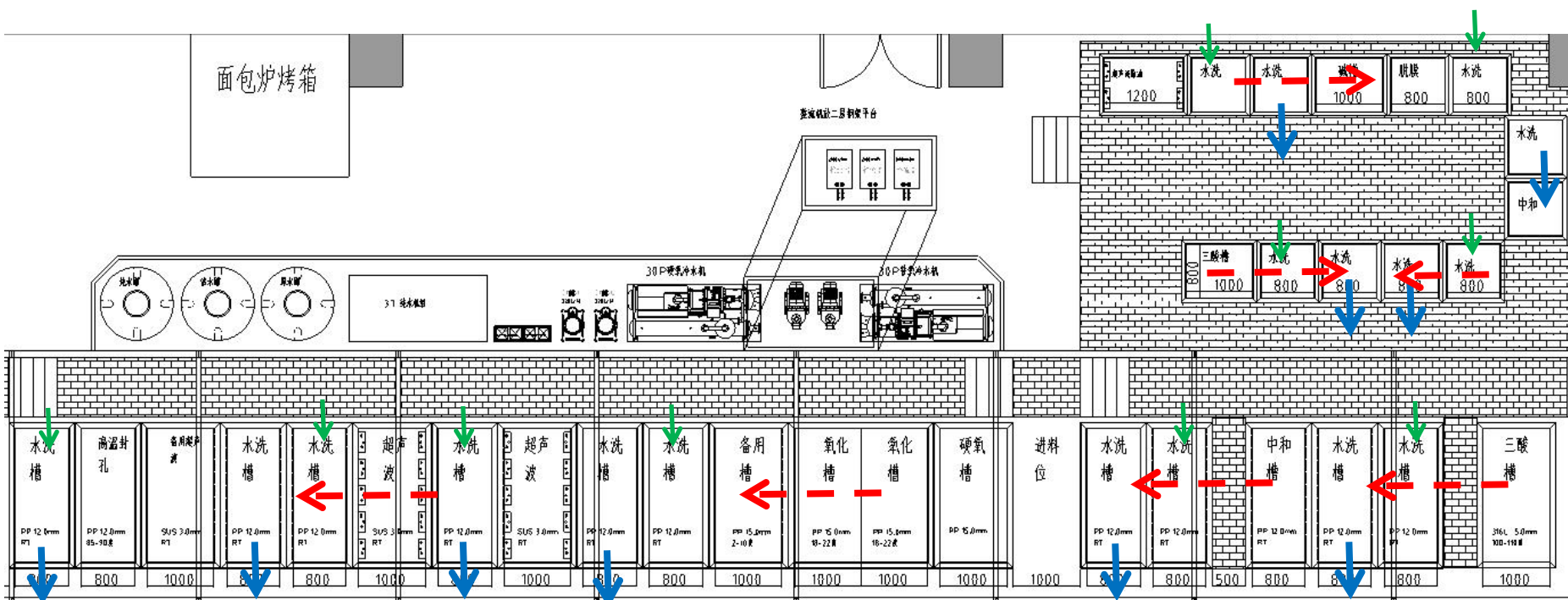
图 4.1-9 1#阳极氧化线槽体连接图 (1)
