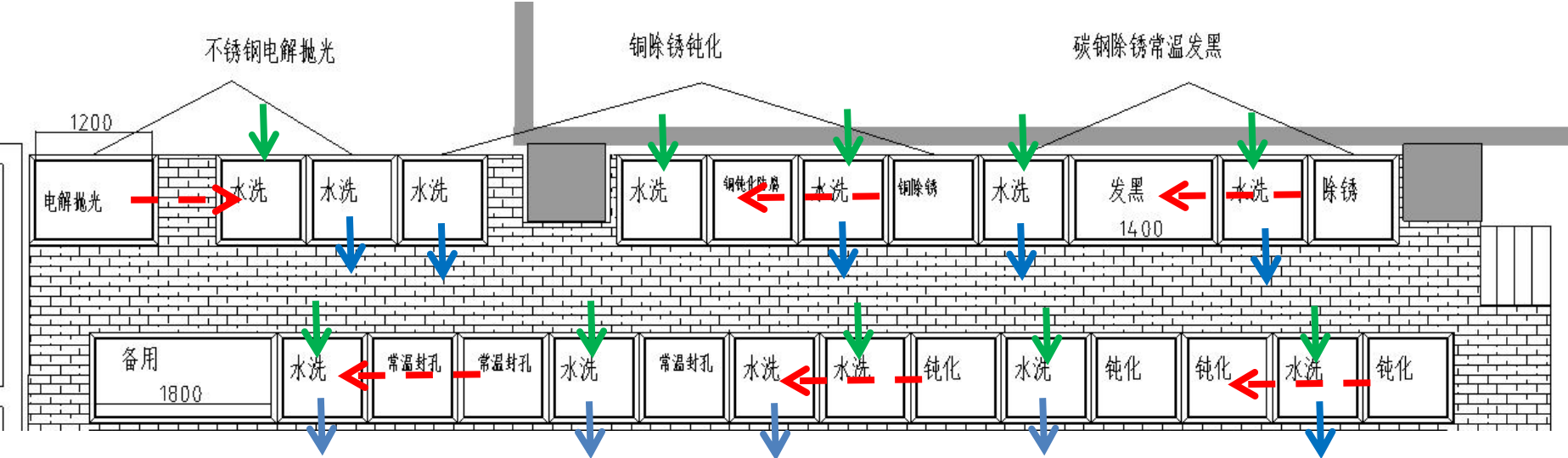
图 4.1-8 不锈钢件、铜件、铁件表面处理槽体连接图
