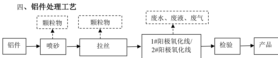
图 4.1-4 项目生产工艺流程图
