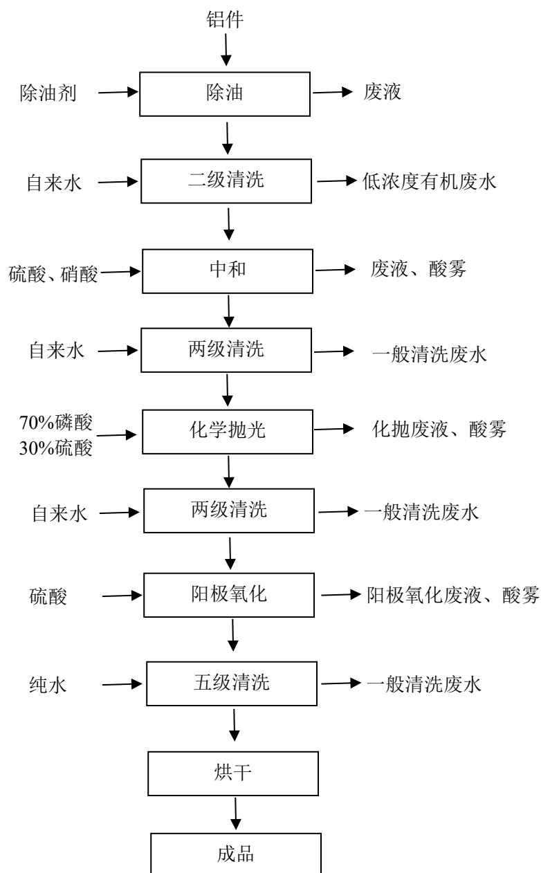
图 4.1-6 2#阳极氧化线工艺流程及产污环节图
