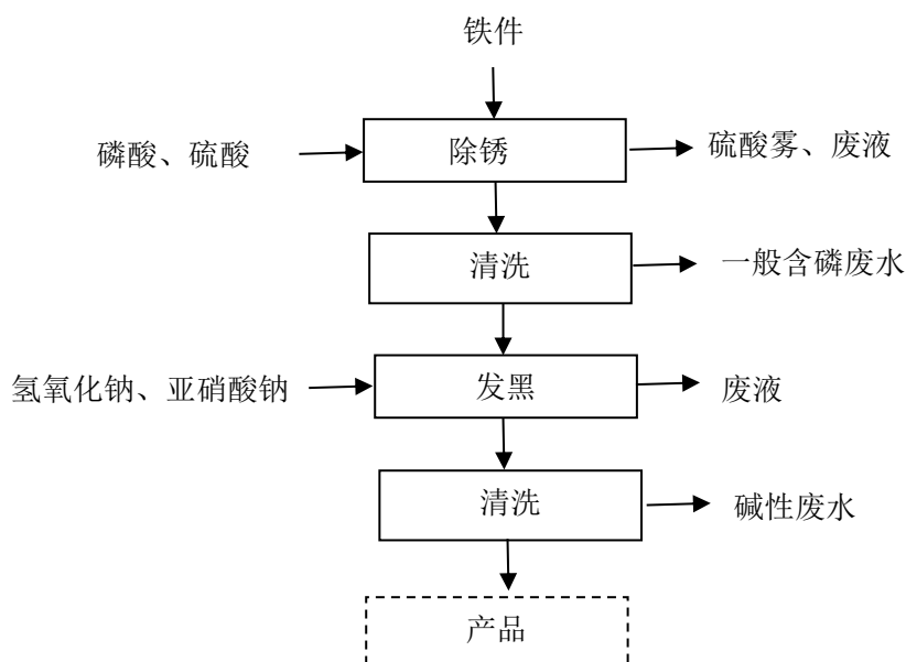
图 4.1-3 铁件表面处理流程及产污环节图
