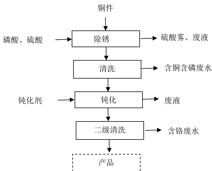
图 4.1-2 铜件表面处理流程及产污环节图
