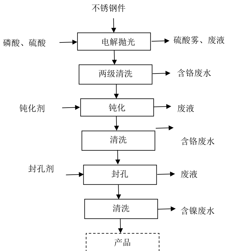
图 4.1-1 不锈钢件表面处理流程及产污环节图
